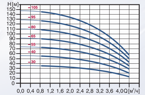
SQ 3 / SQE 3
