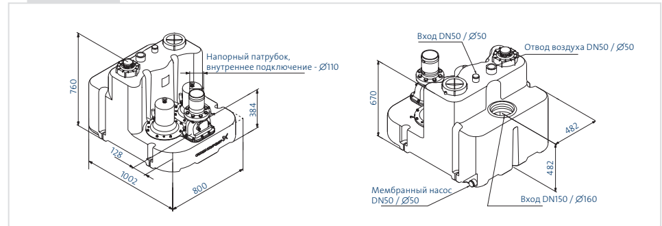
MULTILIFT MLD
