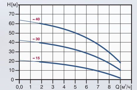
SQ 7 / SQE 7
