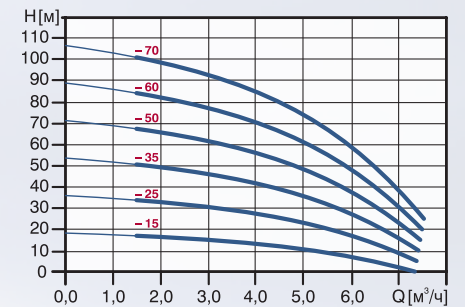
SQ 5 / SQE 5
