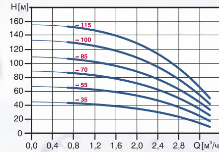
SQ 2 / SQE 2
