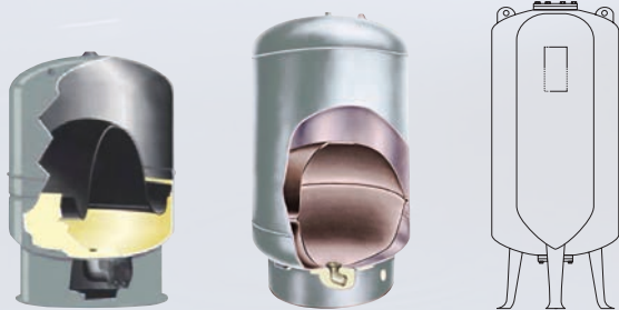
GT-H – одинарная мембрана GT-D – двойная мембрана GT-U – мембрана в виде "груши"
